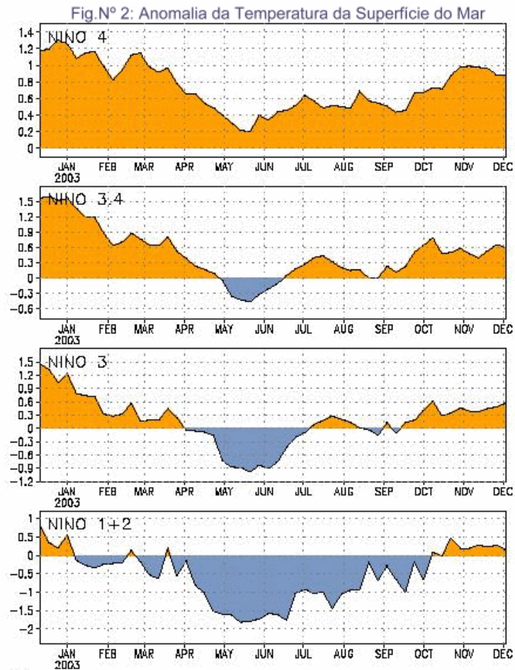
Anomalias da temperatura da superfície da água do Oceano Pacífico Equatorial (baseadas na média de 1950 a 1977), medidas em vários pontos do oceano durante janeiro e dezembro de 2003.
